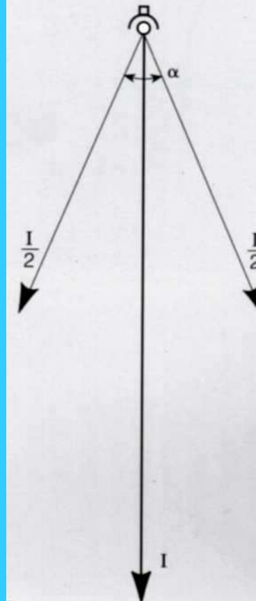
Fig. 25: Convenção da abertura de fecho luminoso de produtos OSRAM.
